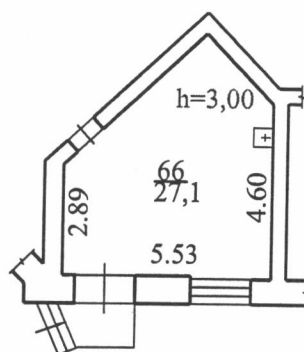
Схема расположения помещения
